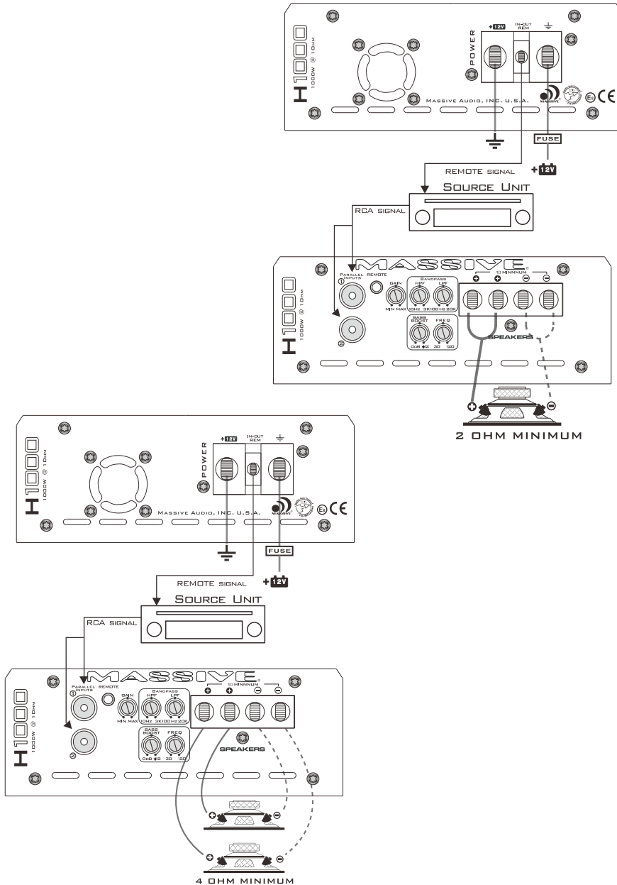
FIG 3. MONO AMPLIFIER WIRING H1000
