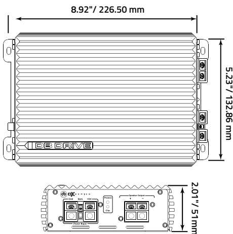
DX-A1201 Dimensions
