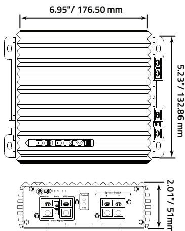
DX-A601 Dimensions
