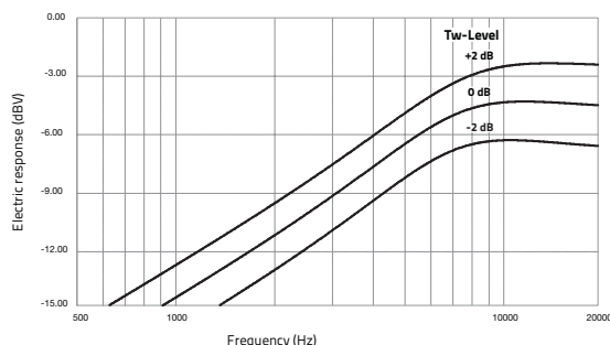
MLCX 165.3: Tweeter-Level
