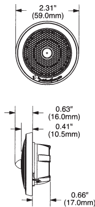
Tweeter
